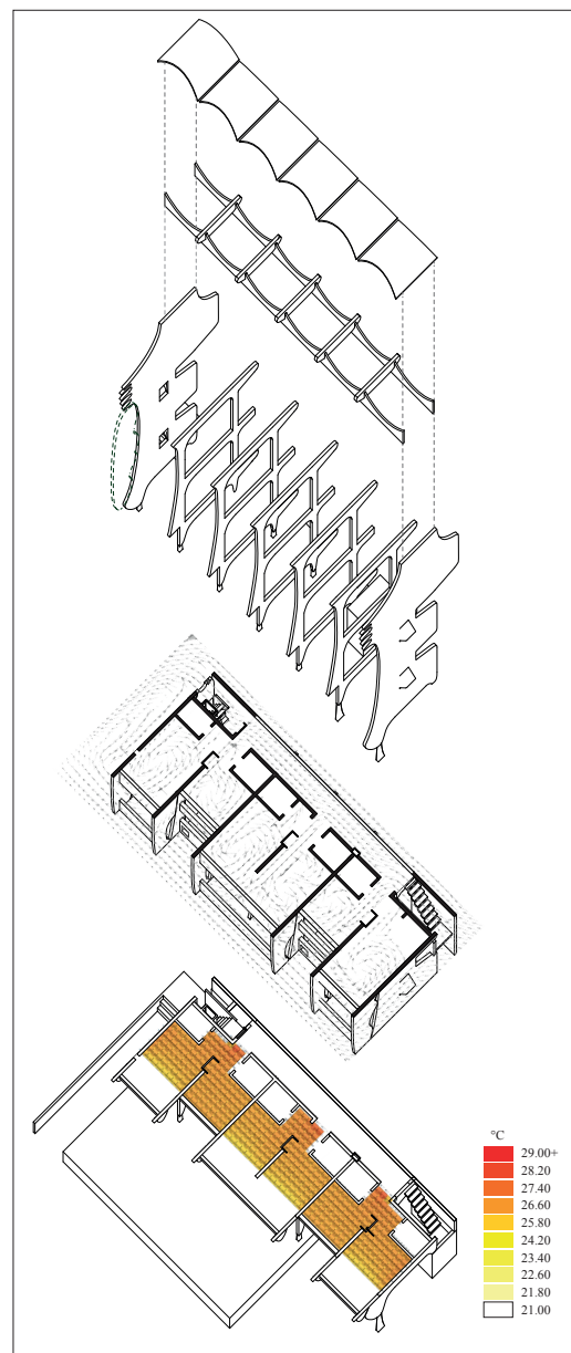
P. Guedes, edificio per appartamenti "Leão que ri" [Leone sorridente], Lourenço Marques 1955-1958. In alto: disegni di archivio A lato: Le ragioni della forma: tecniche (calcestruzzo armato) e mitigazione del clima (raffrescamento e tempertu- re interne). Studi e disegni di S. Murgia (2023). ©Archivio Guedes ©SamueleMurgia
